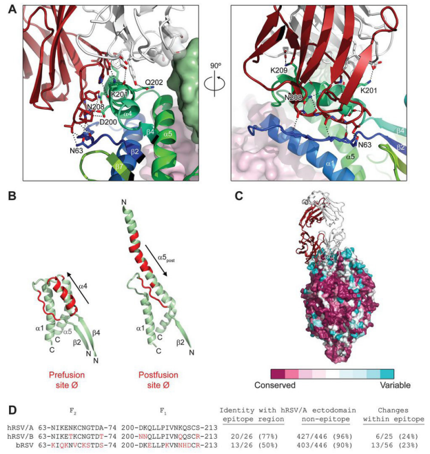
Рисунок 17 | Взаимодействие F-белка респираторно-синцитиального вируса с антителом D25. Антитело связывается с эпитопом, включающем в себя 2 протомера на верхушке префузионного F-белка. Красным цветом обозначены атомы кислорода, синим - атомы азота
